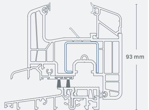
Barrier-free balcony door threshold Fig.: 1:2
